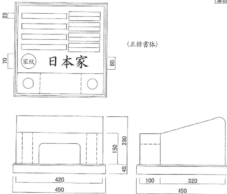
墓石部図面
